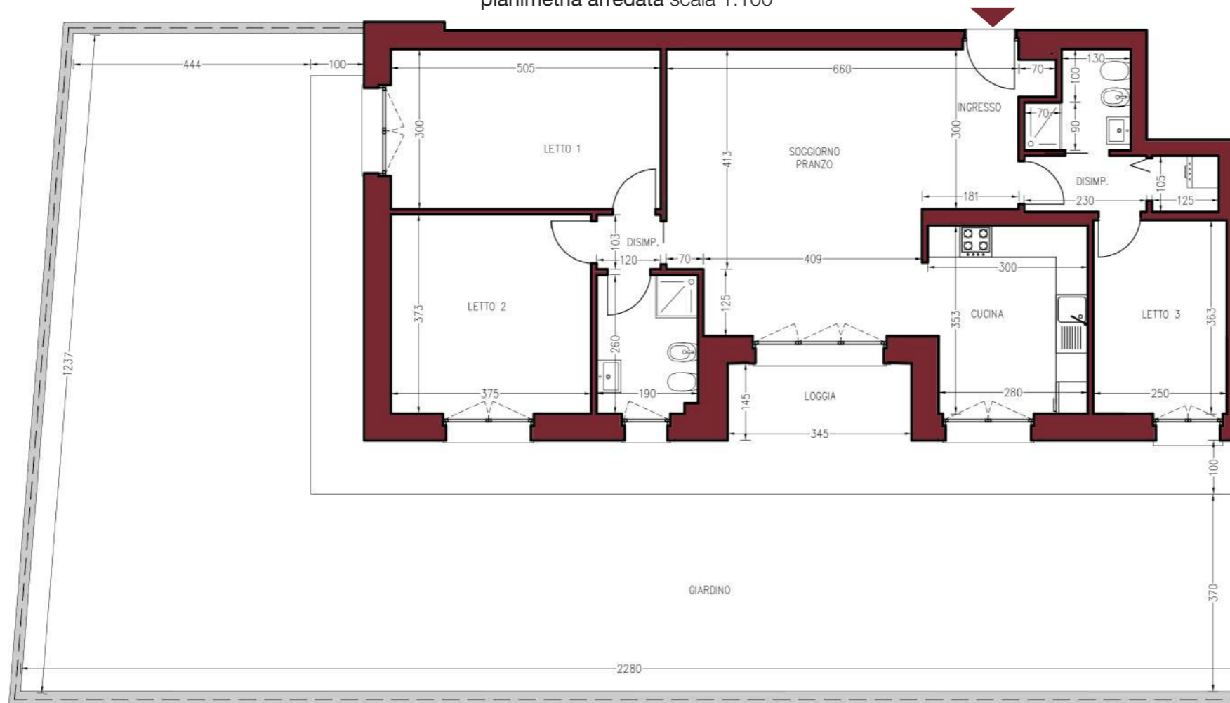
planimetria quotata scala 1:100
